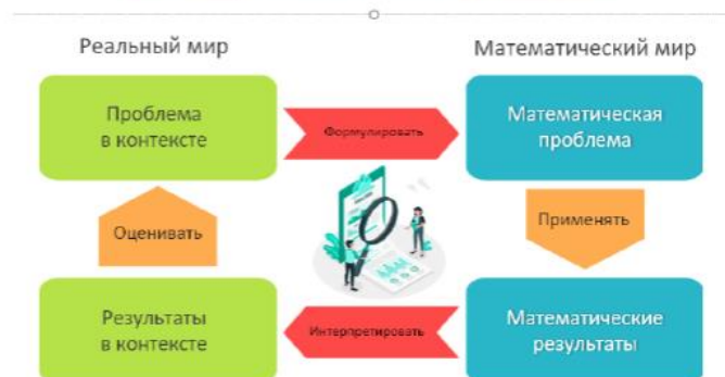
Рис. 1. Диагностическая модель математической грамотности
